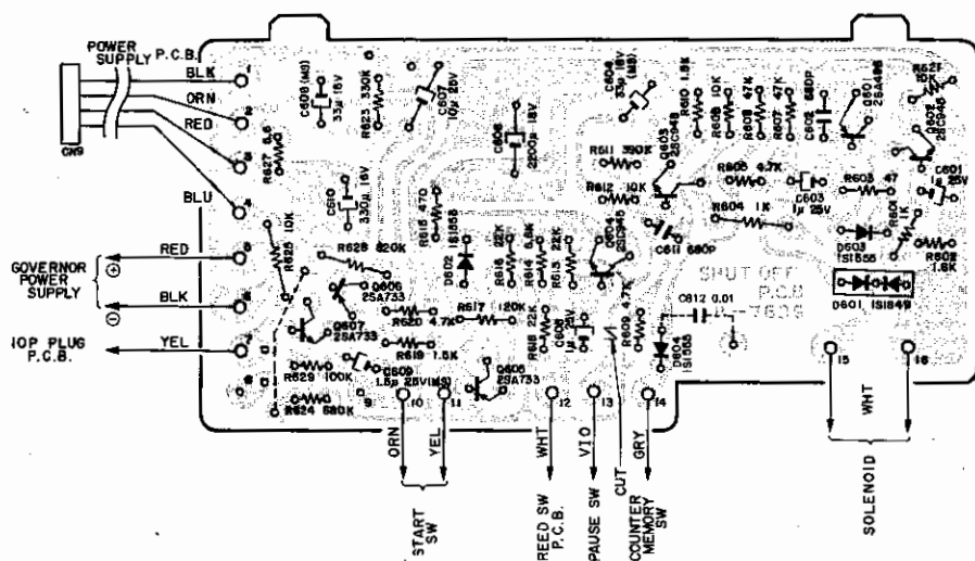
Fig. 8.9.1 (Serial No. 3811501-)
