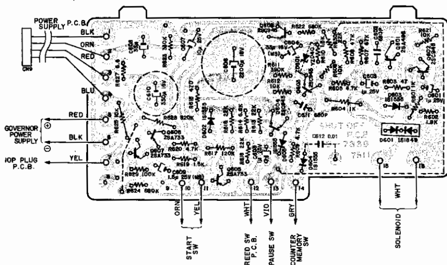
Fig. 8.9.1 (Serial No. 3811501-)
